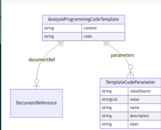
ER Diagram: AnalysisProgrammingCodeTemplate
